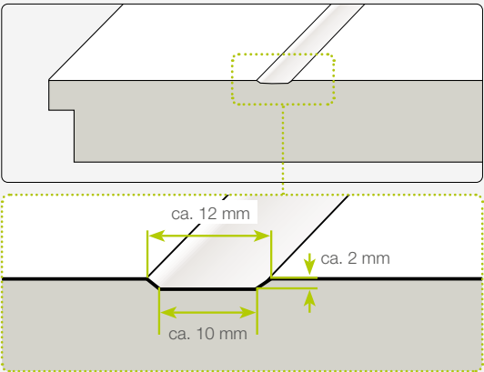
Lines Art | Querschnitt
