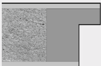
2 ECKIGE KANTE (EC) CHANT CARREE (EC)
