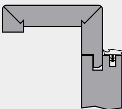
4 ZARGE MIT KLEINER RUNDKANTE CADRE AVEC PETIT CHANT ARRONDIS
